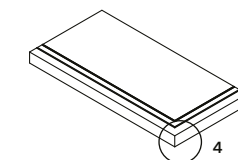
step extra thick corner inox* nez de marche forte épaisseur angle inox* ecke massive stufenplatte inox* degrau espessurado canto inox* 30x89 . 12"x35" P MP-6690 30x90 . 12"x36" SM MP-6690 30x120 . 12"x48" SM . P MP-6710
